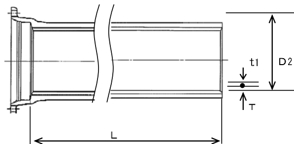
ダクティル鉄管K形寸法表
